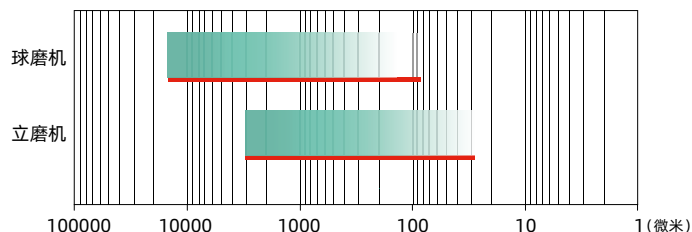
球磨机和立磨机的一般应用范围（微米）
